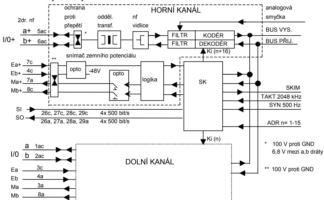
Obrázek č. 2 Blokové schéma jednotky EM2P
