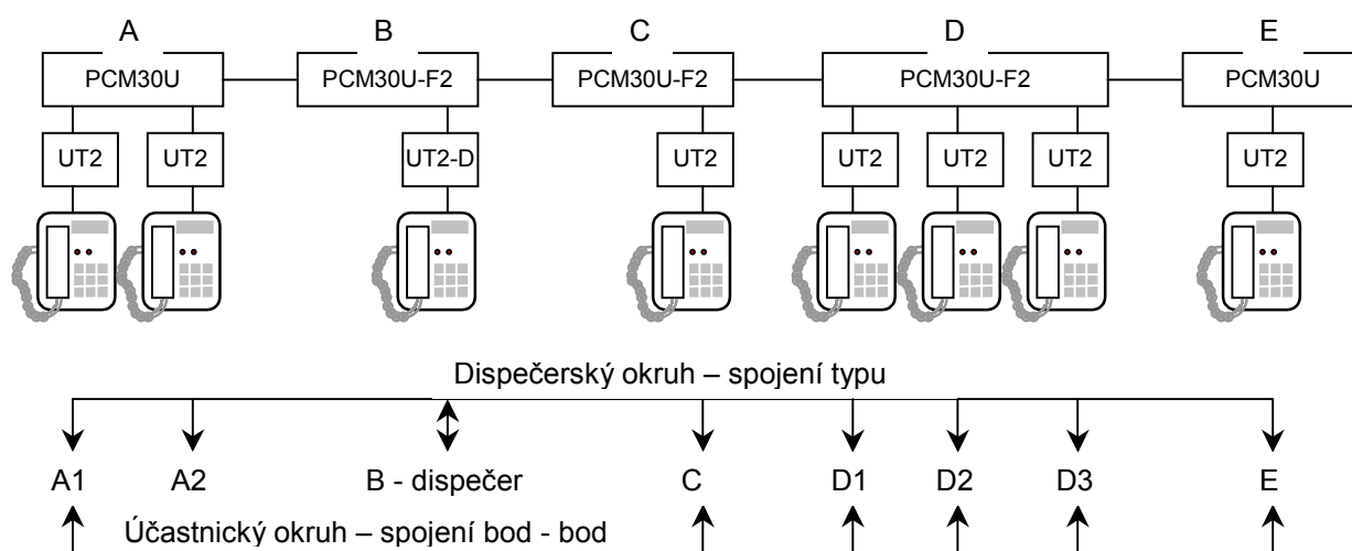
Obrázek č. 11 Možnost zapojení jednotky UT
