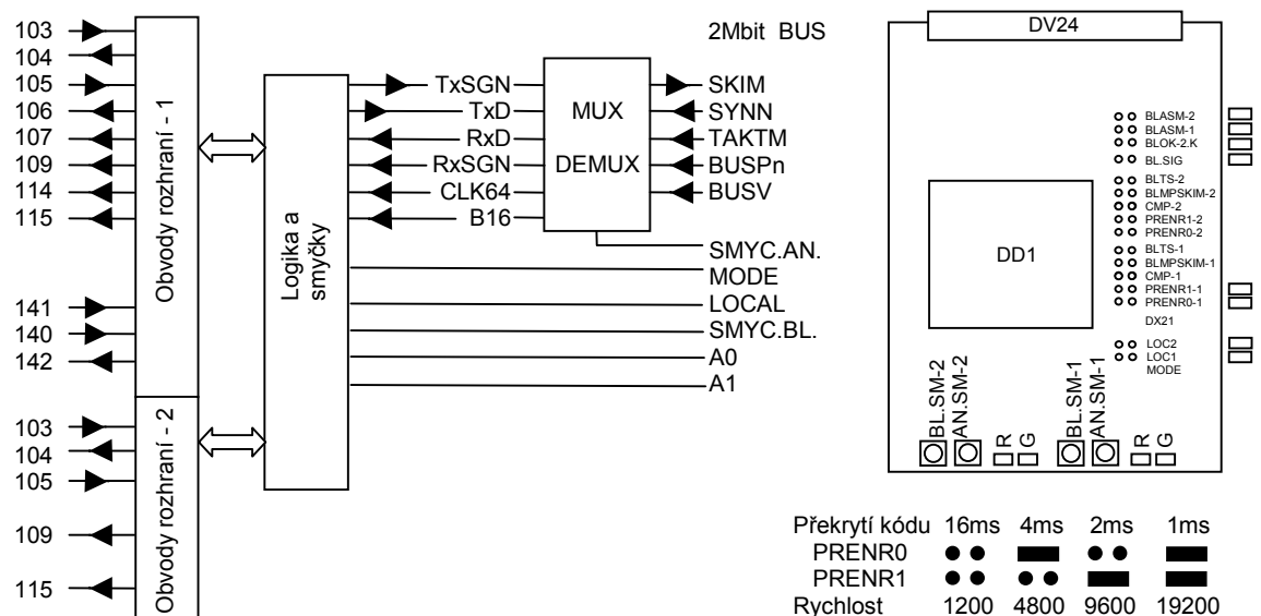
Obrázek č. 28 Blokové schéma jednotky DV24
