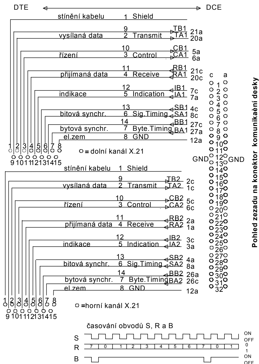
Obrázek č. 23 Příklad připojení fyzické vrstvy rozhraní X.21 jednotky DX21 na konektor komunikační desky rámu PCM30U
