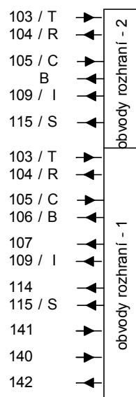
Obrázek č. 21 Blokové schéma a nastavovací prvky jednotky DX21
