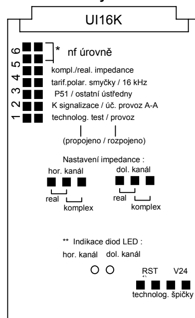
Obrázek č. 8 Možnosti nastavení jednotky UI16K
