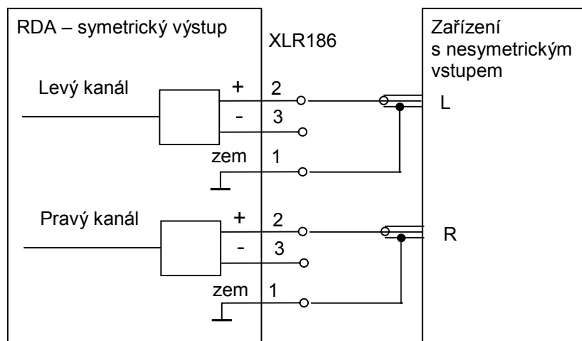
Obrázek č. 47 Připojení zařízení s nesymetrickým vstupem
