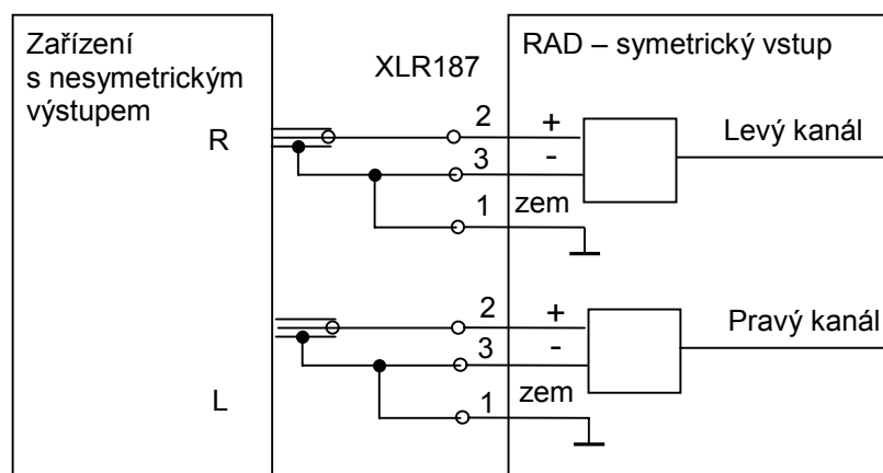
Obrázek č. 45 Připojení zařízení s nesymetrickým výstupem
