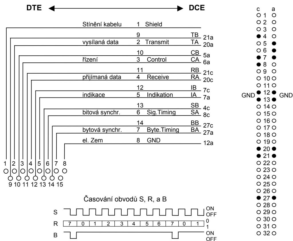
Obrázek č. 35 Připojení rozhraní X21 jednotky RK na konektor
