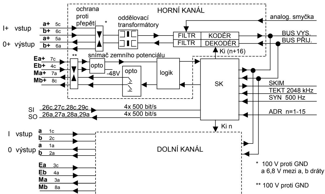
Obrázek č. 4 Blokové schéma jednotky EM4P
