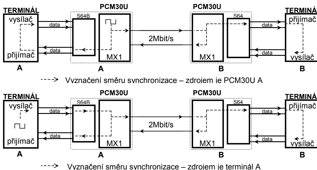
Obrázek č. 18 Schéma šíření synchronizace jednotky S64
