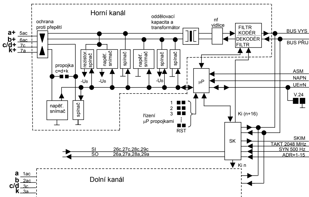
Obrázek č. 15 Blokové schéma jednotky KPR2
