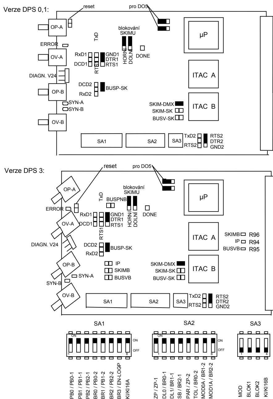
Obrázek č. 41 Rozmístění nastavovacích a signalizačních prvků na DO1
