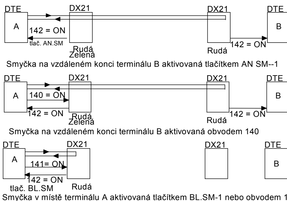
Obrázek č. 22 Aktivace smyček jednotky DX21
