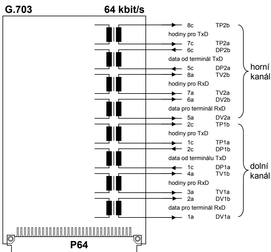
Obrázek č. 17 Vstupy a výstupy jednotky P64
