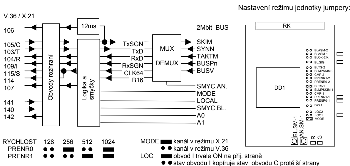
Obrázek č. 34 Blokové schéma jednotky RK
