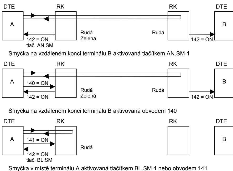
Obrázek č. 36 Funkce smyček u jednotek RK
