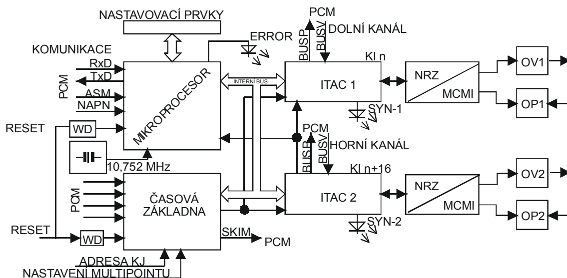
Obrázek č. 40 Blokové schéma jednotky DO1
