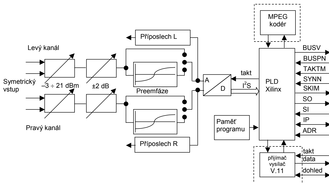
Obrázek č. 44 Blokové schéma RAD
