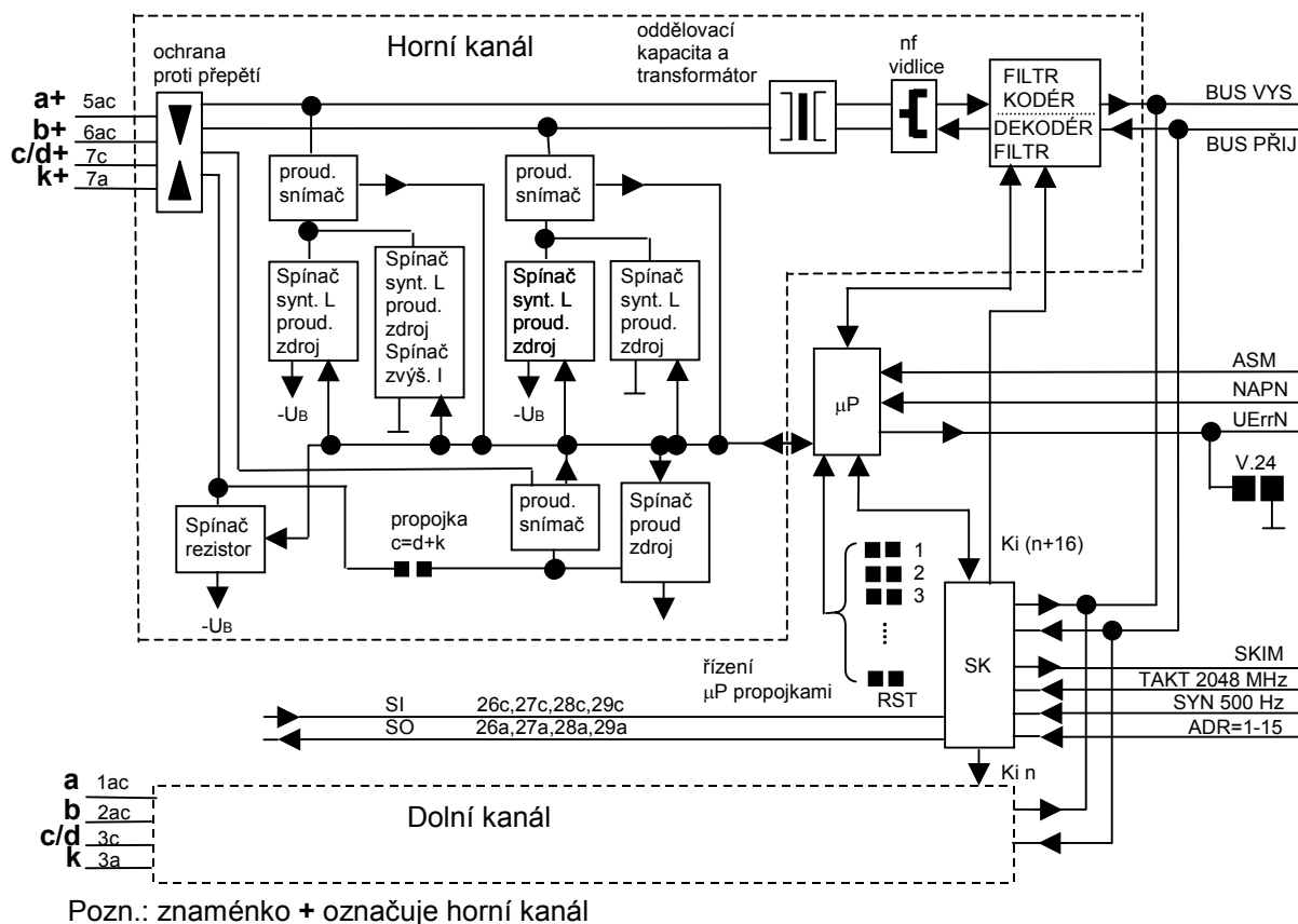
Obrázek č. 14 Blokové schéma jednotka PKR2
