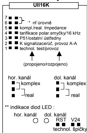
Obrázek č. 10 Možnosti nastavení jednotky U116K
