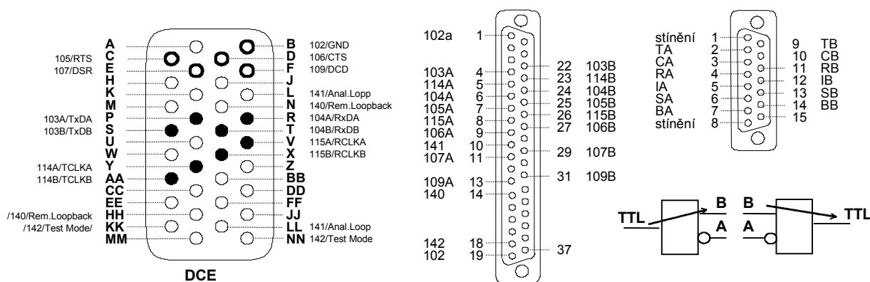
Obrázek č. 39 Příklady použitých konektorů D-SUB pro jednotku RK
