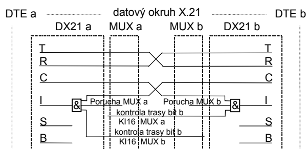
Obrázek č. 24 Připojení datových okruhů u jednotky DX21
