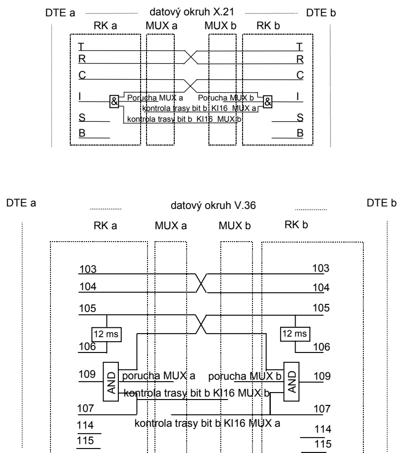
Obrázek č. 37 Připojení jednotky RK podle doporučení ITU-T
