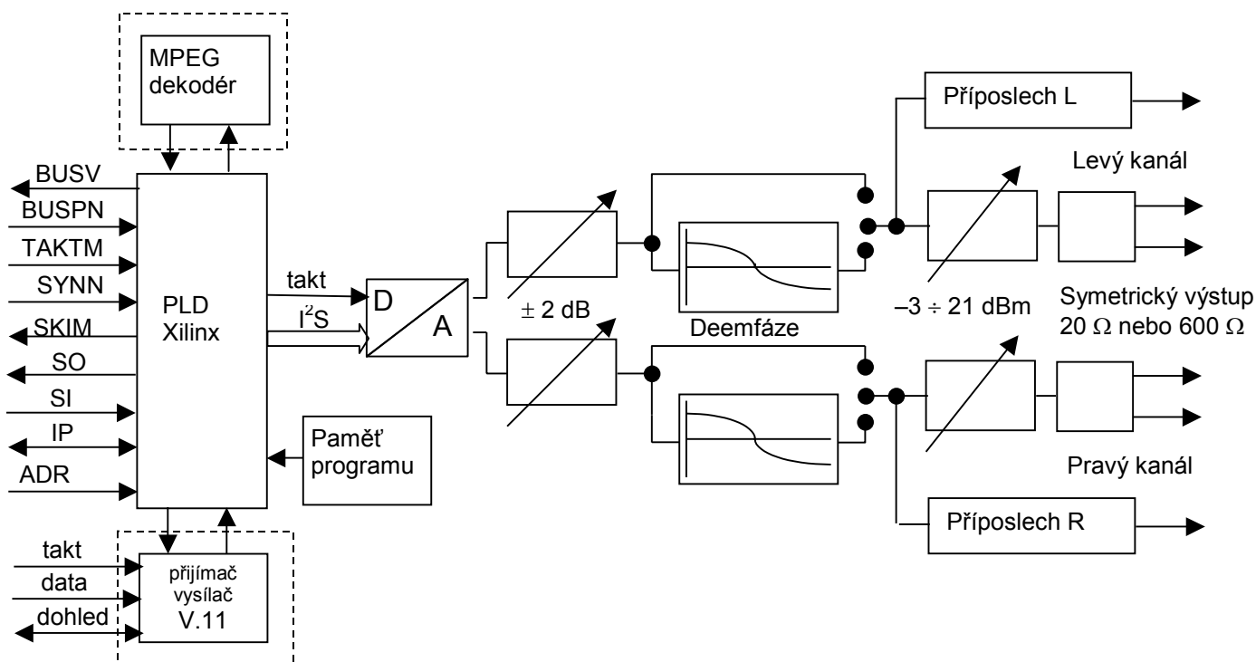
Obrázek č. 46 Blokové schéma
