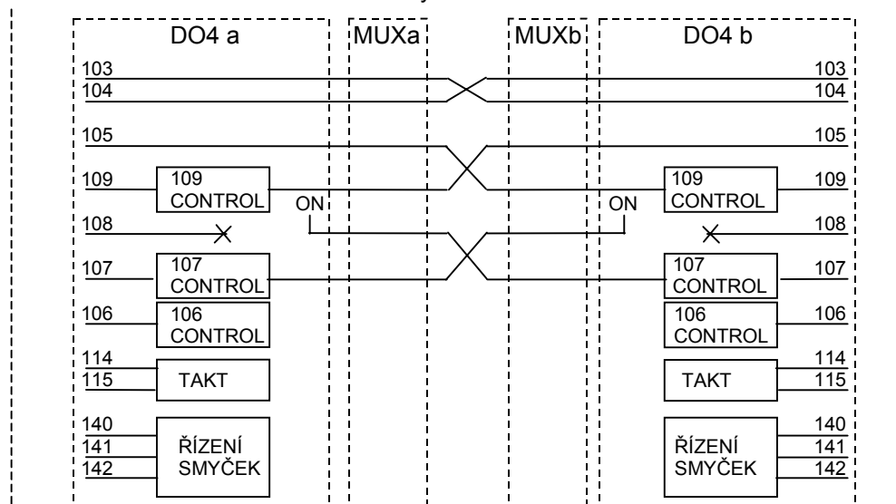
Obrázek č. 43 Připojení jednotky DO4 na datové rozhraní V.24/V.28 dle doporučení ITU-T
