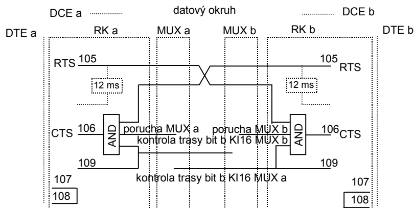
Obrázek č. 38 Připojení jednotky RK na datová rozhraní
