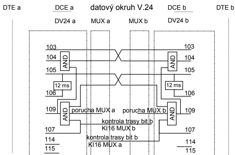
Obrázek č. 30 Připojení a funkce propojení jednotky DV24
